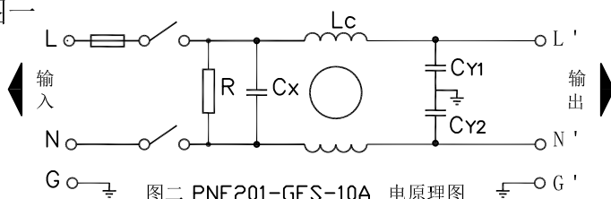
图二 PNF201-GFS-10A 电原理图
