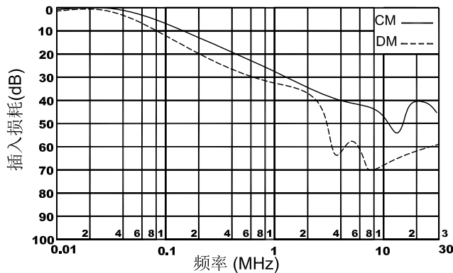
图三 PNF201-GFS-10A 插入损耗曲线图
